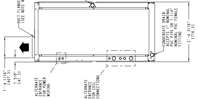
Fig. 2 - Dimensions - 12.5 - 20 Ton Units
