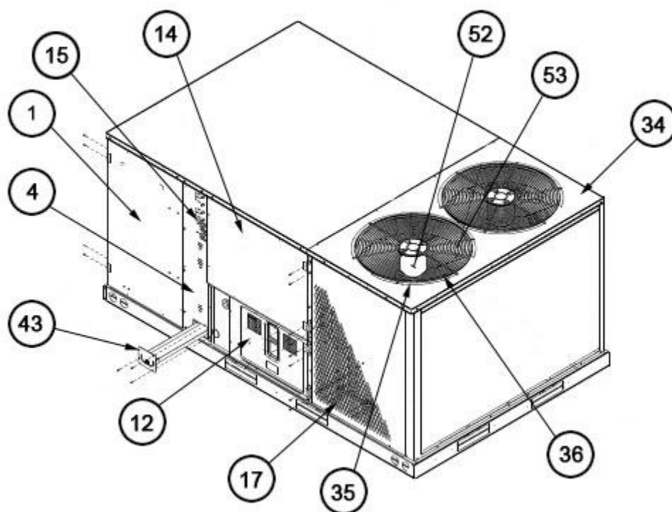
Exterior - Front 090-151
