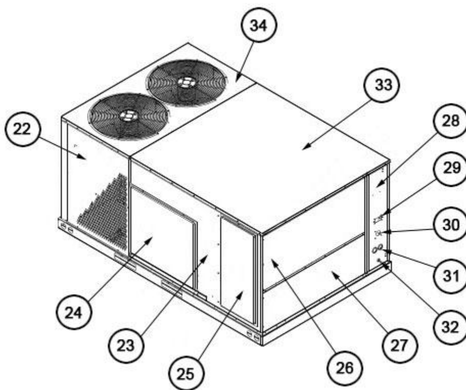
Exterior - Back 090-151
