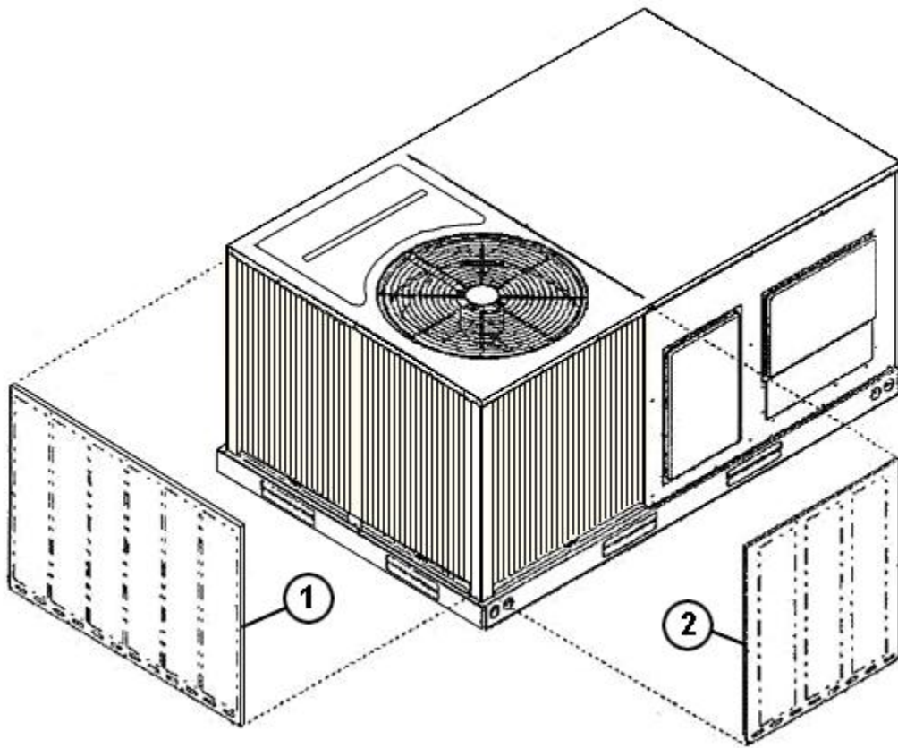
AXRX-AAD02B Assembly
