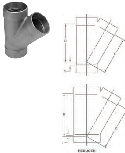
810 \Delta DWV 45° Y C x C x C – Cast
