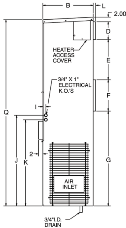
R.H. SIDE VIEW
