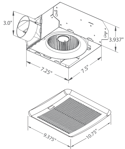
SLM50 Dimensions
